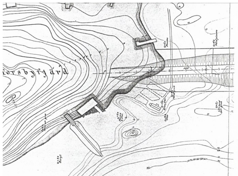
T.h. Kanal genom Ålstäket. Planering 1914 - 1918
