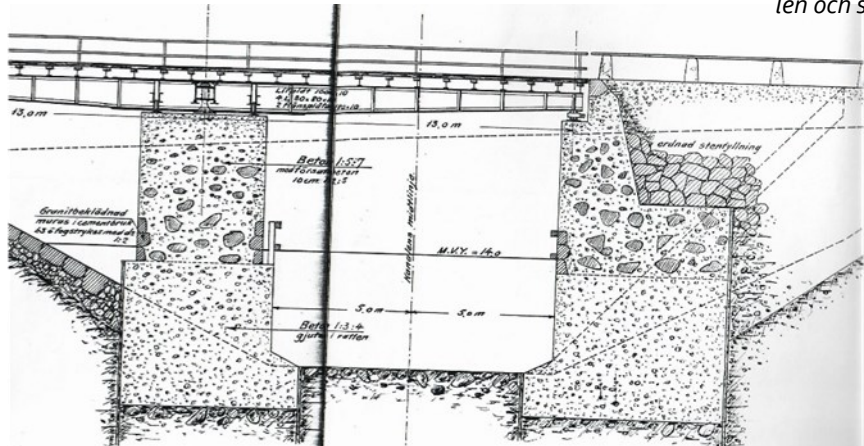
Sektion över kanalen och svängbron.
